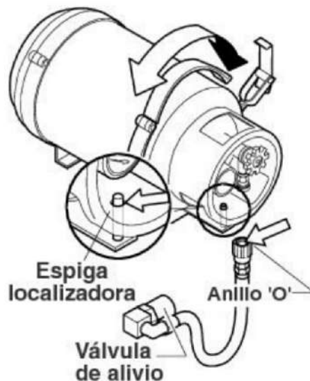
Ilustración de sistema típico
